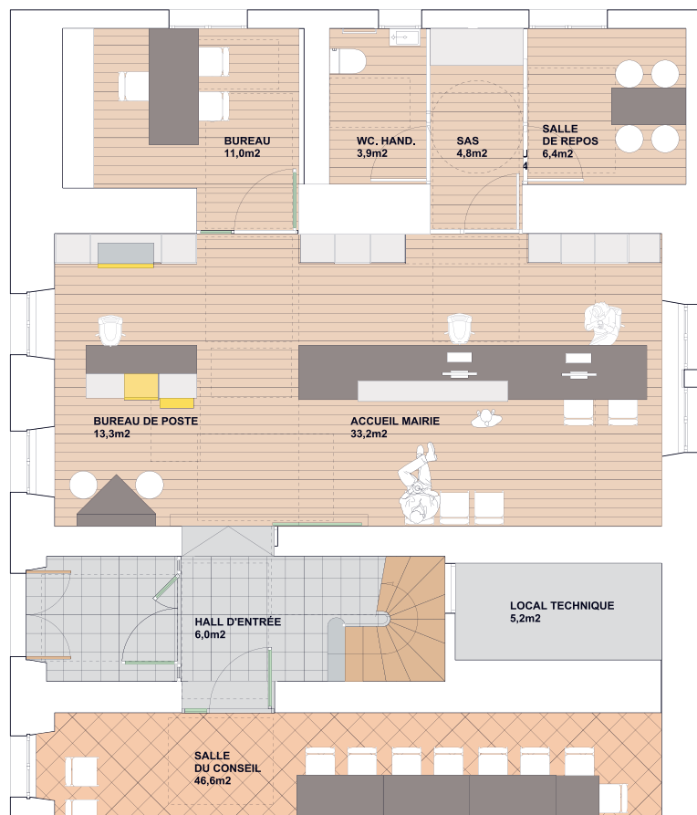
PLAN REZ-DE-CHAUSSEE
